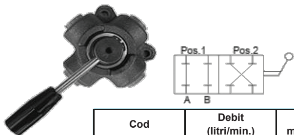
Deviator hidraulic cu 4 căi
