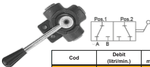
Deviator hidraulic cu 3 căi
