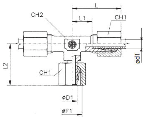
TN120* Adaptor T cu olandeză captivă la mijloc
