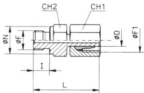
TN126-LM Adaptor drept cu olandeză captivă pe o parte
