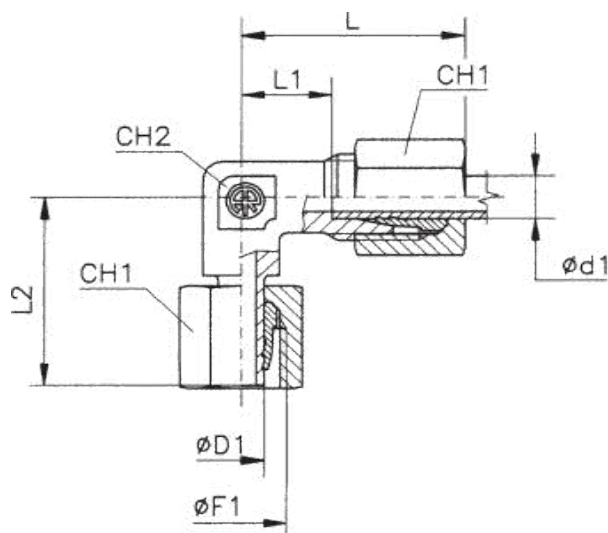
TN119* Adaptor L cu o olandeză captivă
