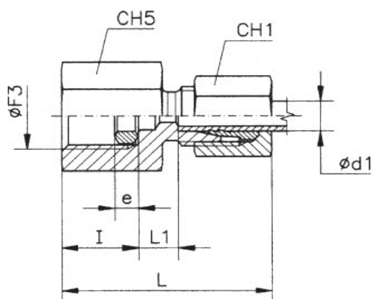
TN103* Adaptor manometru FE (filet exterior)
