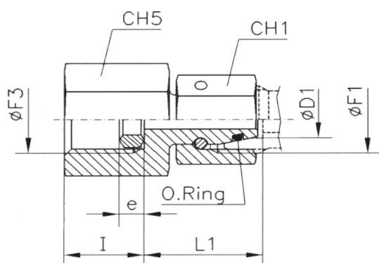
TN403 Adaptor manometru cu olandeză captivă
