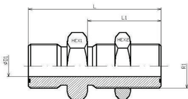
Fiting ORS lung, cu piuliță - FORL
