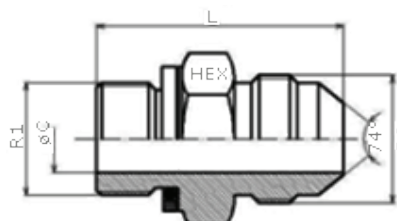
Fiting BSP-UNF - FBZU etanșare dreaptă / con 74 de grade
