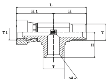
Adaptor BSP T, olandeză lateral - BSPT-FIOL filet interior, cu olandeză / filet exterior / filet exterior con 60 de grade
