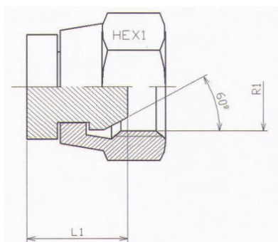
Capac închidere BSP FI - CBSP cu filet interior
