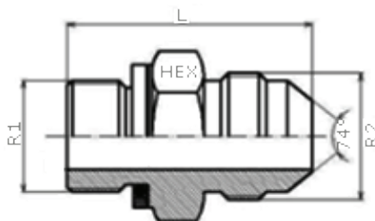
Fiting metric-UNF - FMZU etanșare dreaptă / con 74 de grade
