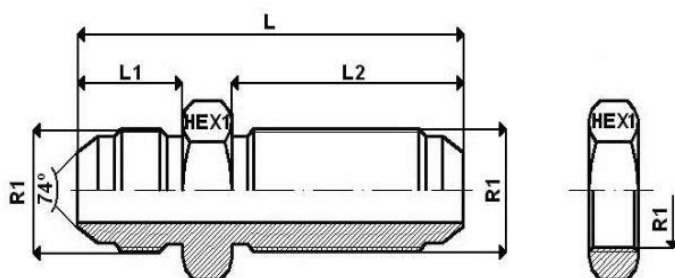
Fiting UNF lung, cu piuliță - FUNFL con 74 de grade
