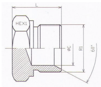
Dop BSP FE - DBSP cu filet exterior
