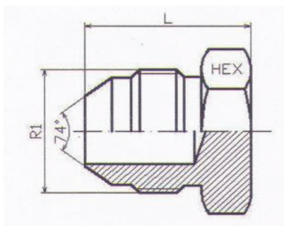
Dop UNF FE - DUNF cu filet exterior
