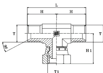
Adaptor BSP T, olandeză mijloc - BSPT-FIOM filet exterior / filet interior, cu olandeză / filet exterior con 60 de grade
