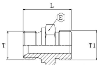
Fiting ORS/metric - FORMZ metric etanșare plană
