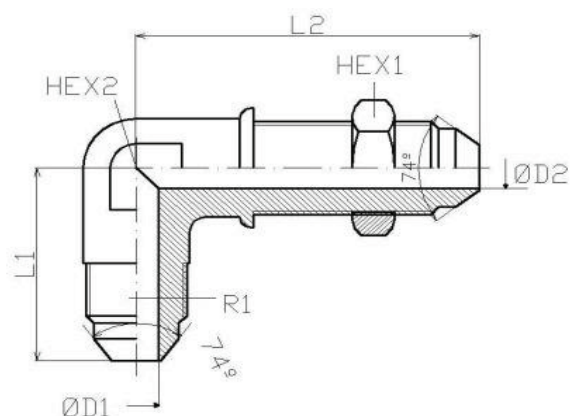
Adaptor UNF L orientabil - UNFL-FEOR filet exterior con 74 de grade
