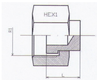
Capac închidere ORFS FI - CORF cu filet interior
