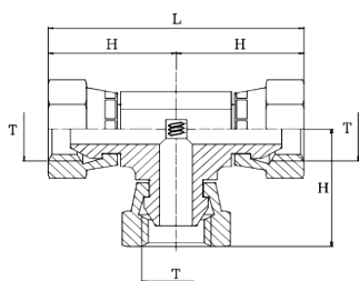
Adaptor BSP T cu olandeze - BSPT-FIO filete interioare, cu olandeze con 60 de grade
