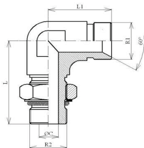
Adaptor BSP L orientabil - BSPL-FEZORFE filet exterior etanșare plană / con 60 de grade
