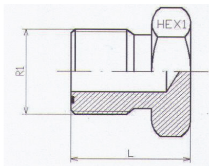
Dop ORFS FE - DORS cu filet exterior
