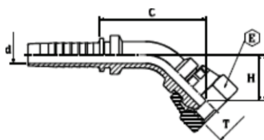
Armătură BSP - DKR45 con 60 de grade
