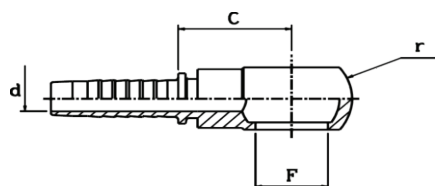
Armătură hidraulică ochi GAS
