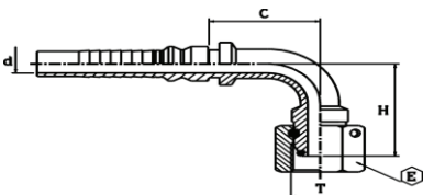
Armătură Interlock BSP - IDKR90 con 60 de grade
