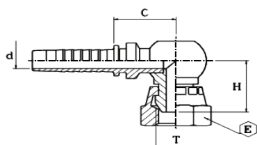
Armătură BSP compact - DKR 90-K con 60 de grade
