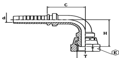
Armătură filet metric - DKM90 con 60 de grade
