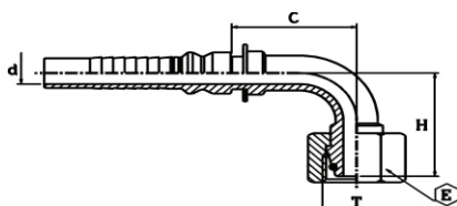
Armătură Interlock cu filet metric - IDKOS90 con 24 de grade
