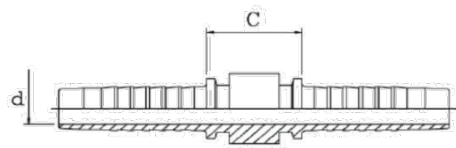
Joncțiune - JONC furtun - furtun
