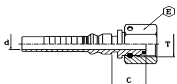
Armătură Interlock BSP - IDKR con 60 de grade
