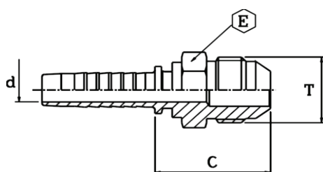
Armătură UNF - AGJ cu filet exterior con 74 de grade
