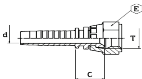
Armătură UNF - DKJ con 74 de grade
