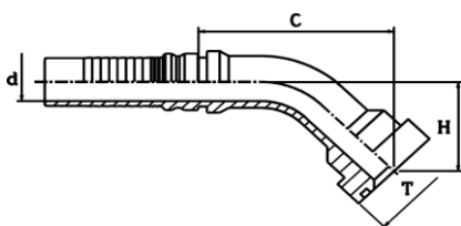
Armătură Interlock flanșă Supercat - IFL45-S
