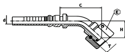
Armătură Interlock BSP - IDKR45 con 60 de grade
