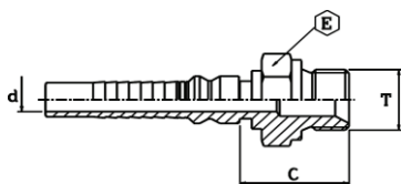
Armătură Interlock BSP - IAGR cu filet exterior con 60 de grade
