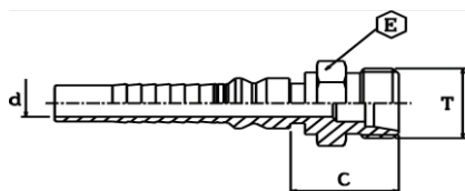
Armătură Interlock cu filet metric exterior - ICES con 24 de grade
