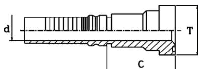
Armătură Interlock flanșă Supercat - IFL-S
