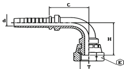
Armătură MULTISEAL, DKL90 DIN 3868 con 24/60 de grade
