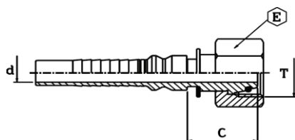
Armătură Interlock cu filet metric - IDKOS con 24 de grade
